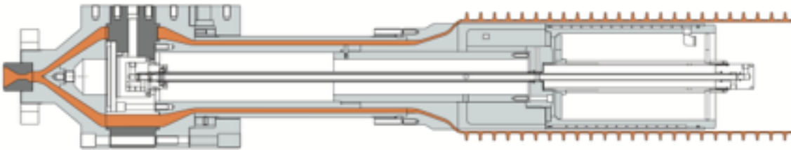
Rib Pipe die.
