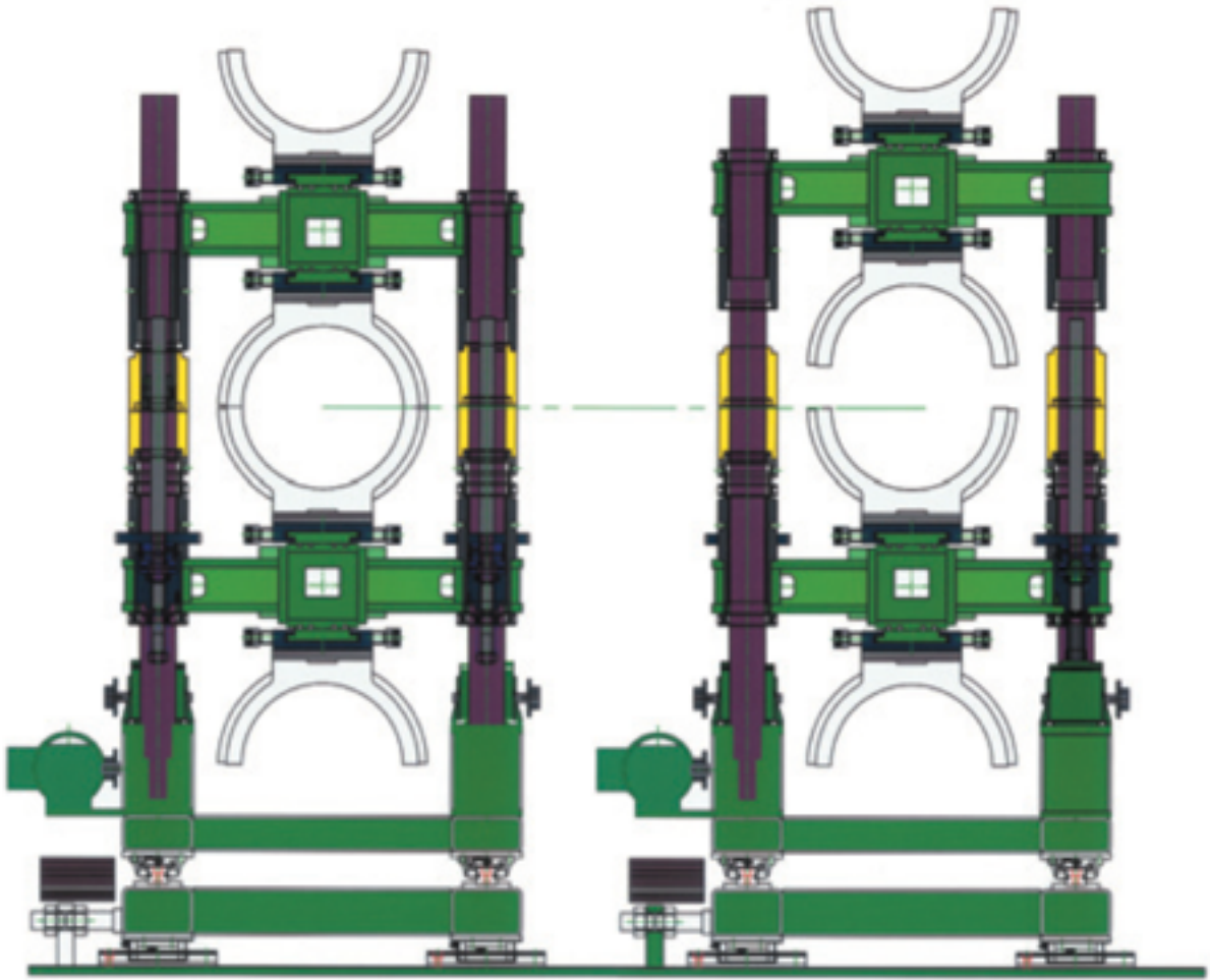
Dikey tasarımlı korugatörlerde üst bölme kaldırma düzeneği ve lineer rulmanlar üzerine yataklanmış sağ-sol ayar mekanizması
